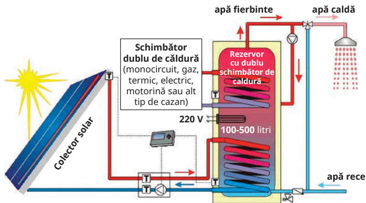
Figura 15. Colectoare solare 16
